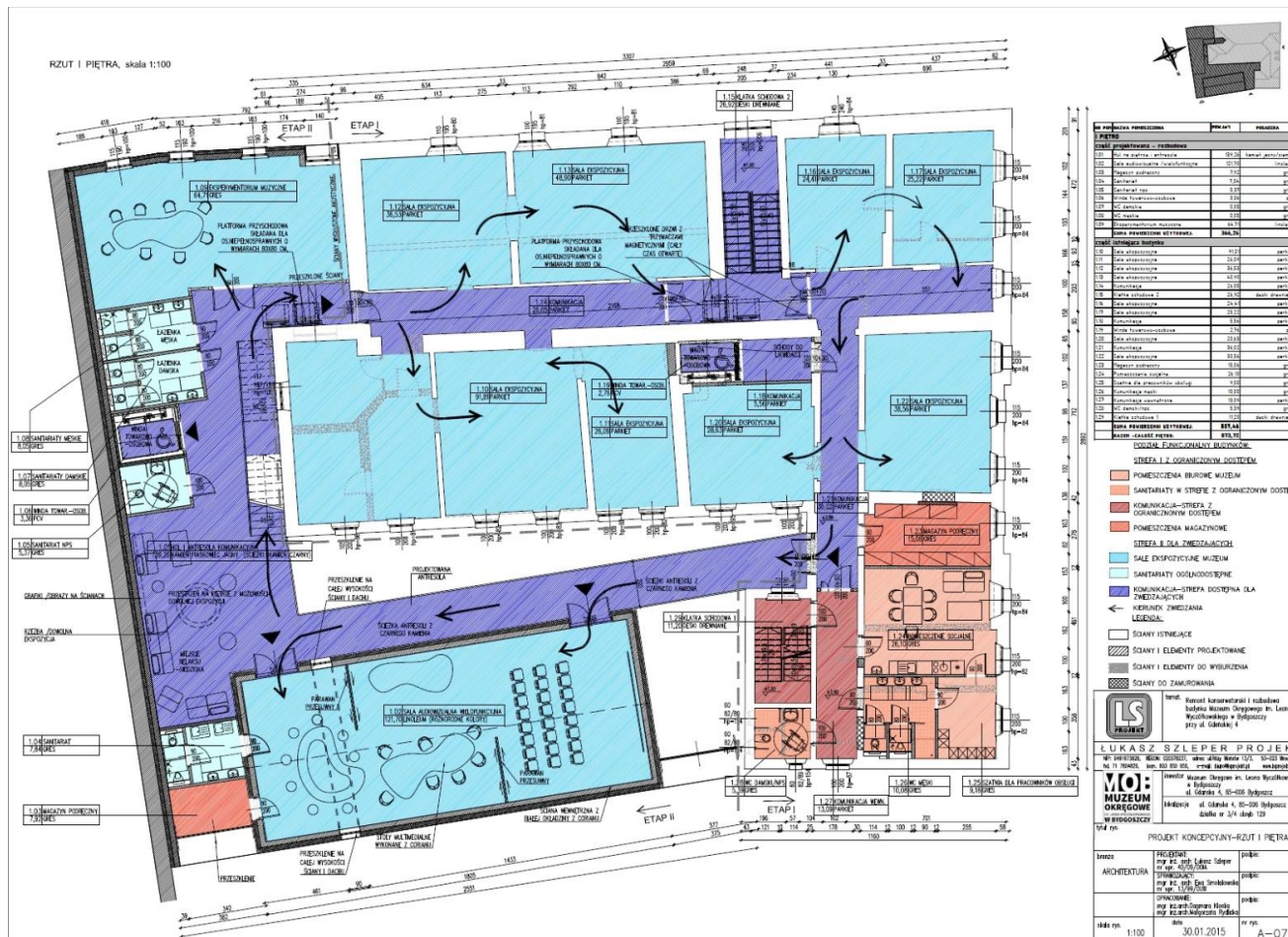
Projekt – rzut I piętra
