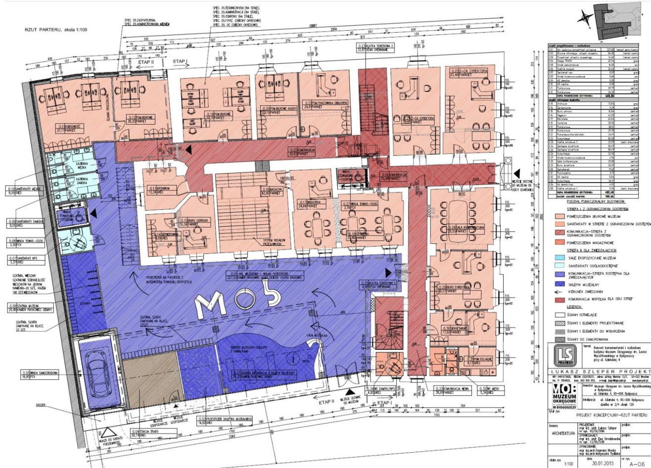
Projekt - rzut parteru
